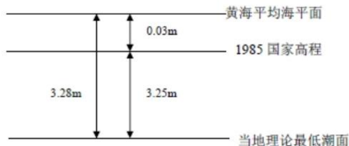
图 5.1-2 基面关系转换图
