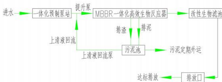
图 6.3-1 沙埕镇污水处理厂工艺流程图
