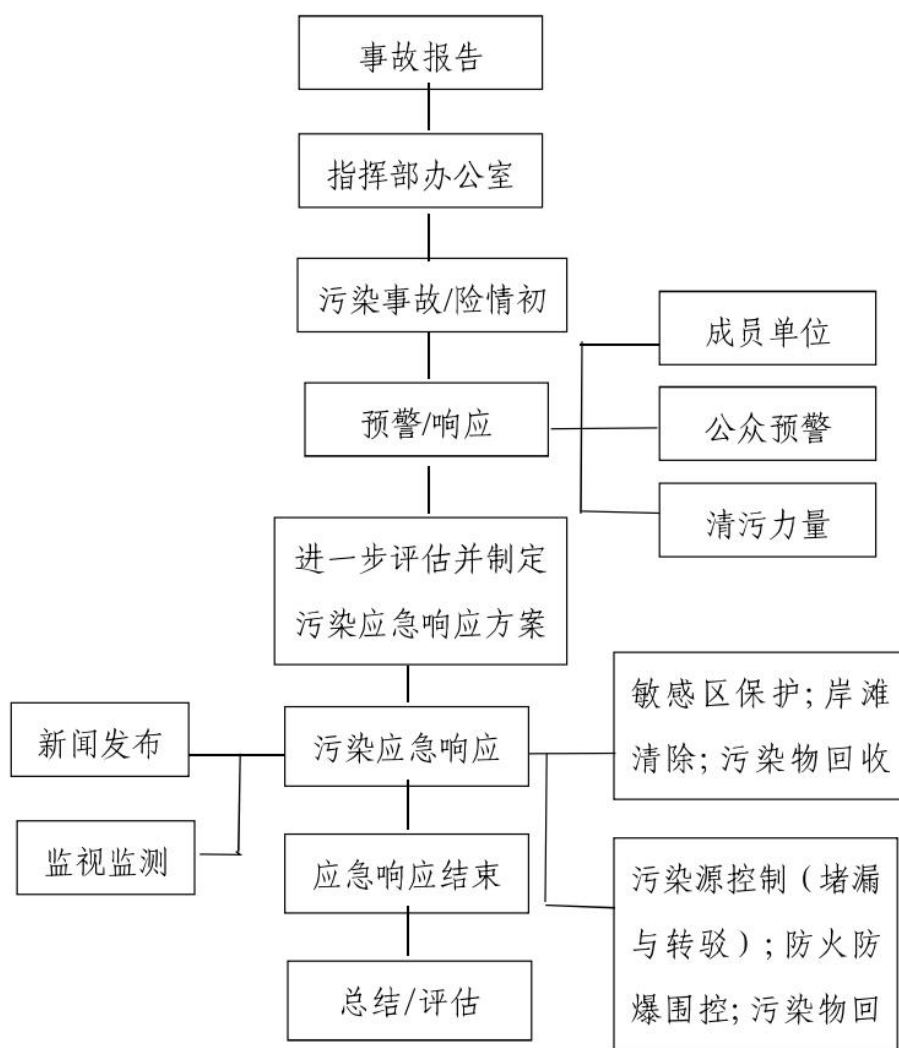
图 7.6-1 宁德海域船舶污染事故应急反应程序图
